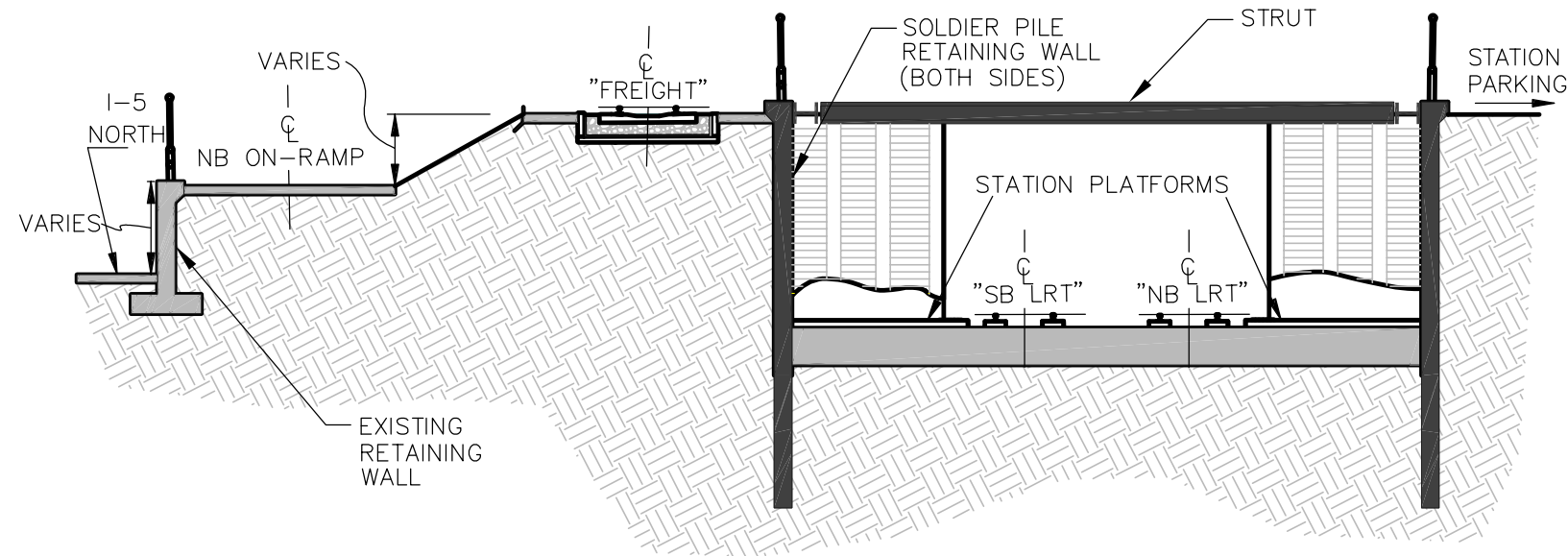
SECTION A-A
